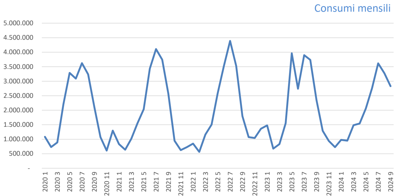
Grafico n. 6 – Consumo mensile in kWh degli impianti negli anni 2020-21-22-23-24
