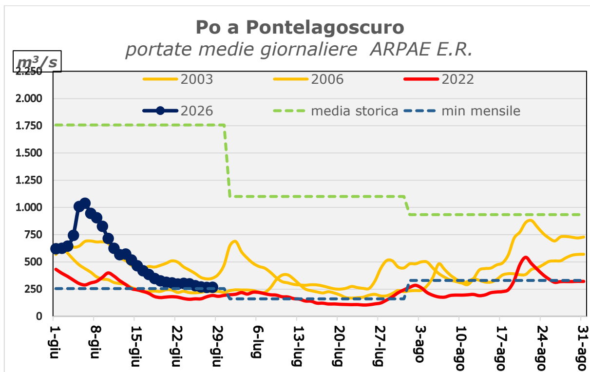
Confronto portate 21-28 giugno a Pontelagoscuro, annualità diverse [mc/sec]
